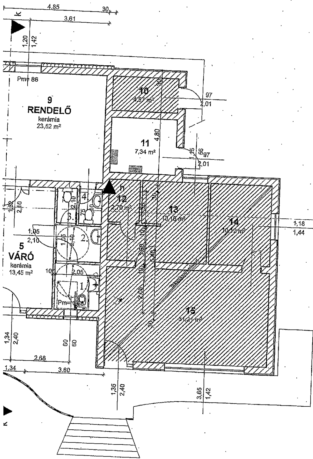
Tervezett alaprajz M=1:100
